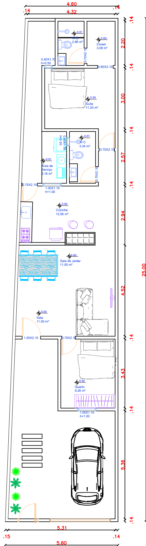
PLANTA BAIXA - TÉRREO Escala 1:100
